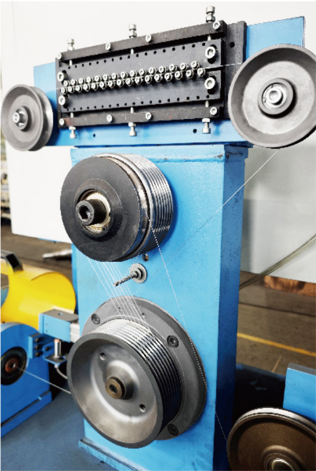
牵引轮+校直器 Traction capstan+straightener
