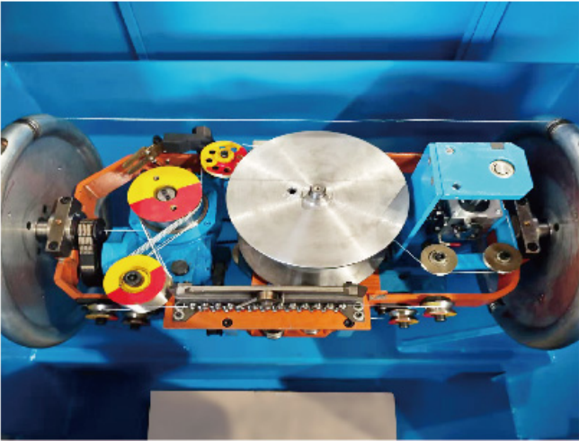
外放内收式收线架 Inner take-up cradle
