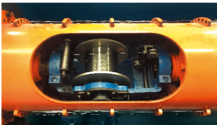
工字轮 Bobbin
